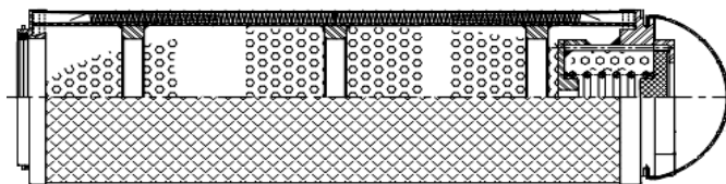
FILTRO HIDRÁULICO RETORNO COM VÁLVULA BY-PASS
